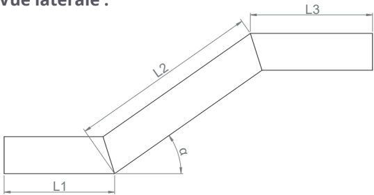
Vue latérale :
